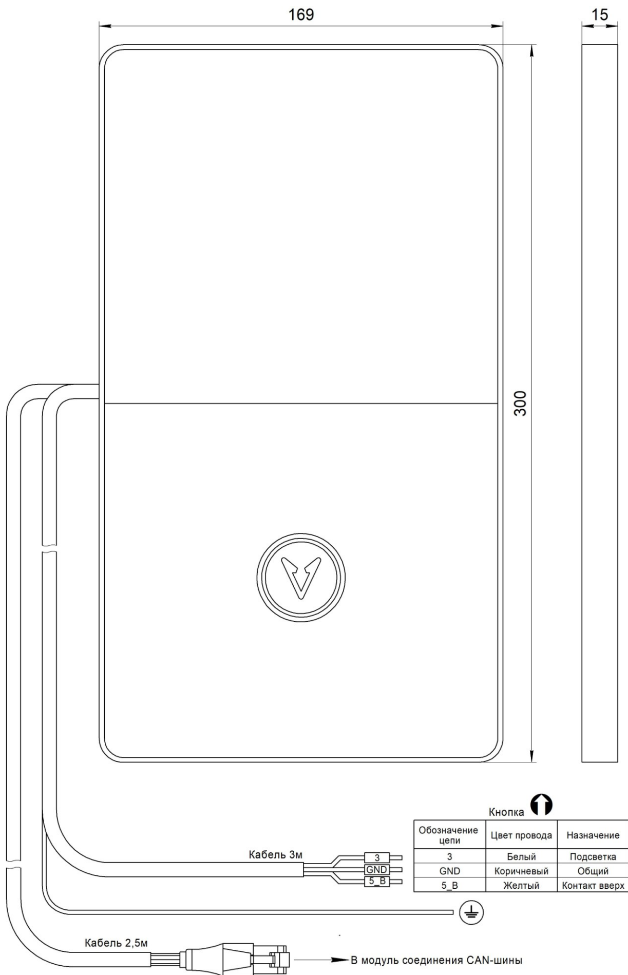
Рис.1 Внешний вид Вызывной пост ОНИКС (жгут RJ45) НШЕК.468381.023-01
